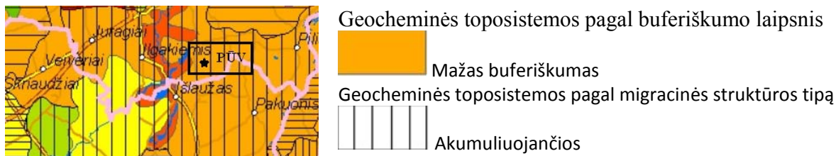
21 pav. Geocheminė toposistema
